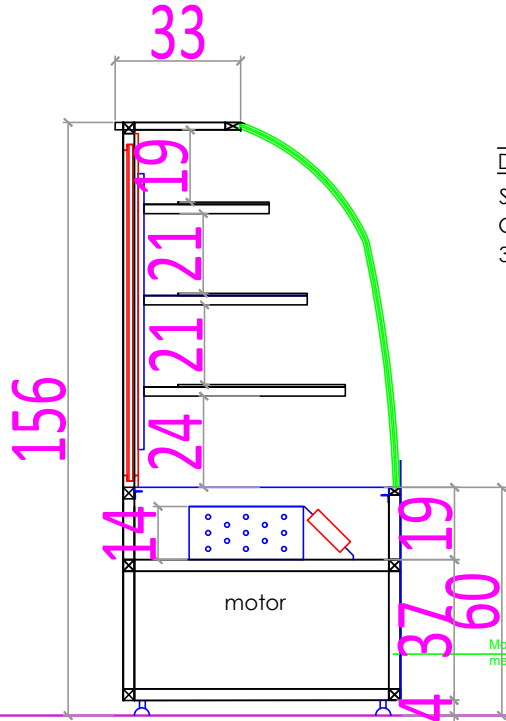
YAN KESİT
